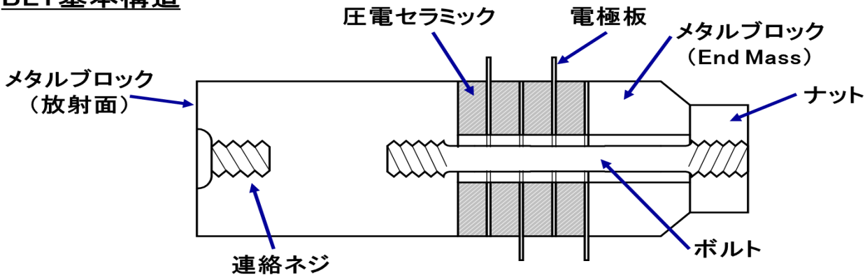
BLT基本構造
